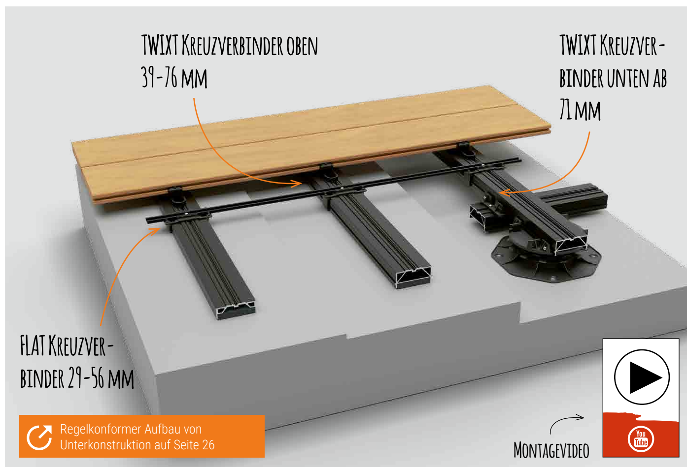
TWIXT Kreuzverbinder unten (ab 71 mm) auf die ausgerichtete Konterlattung einklicken. Aluminium-Unterkonstruktion auf TWIXT Kreuzverbinder unten (ab 71 mm) aufklicken.
